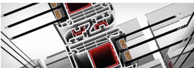
Tetningslister i velur på innsiden, EPDM- og børstelister på utsiden.
